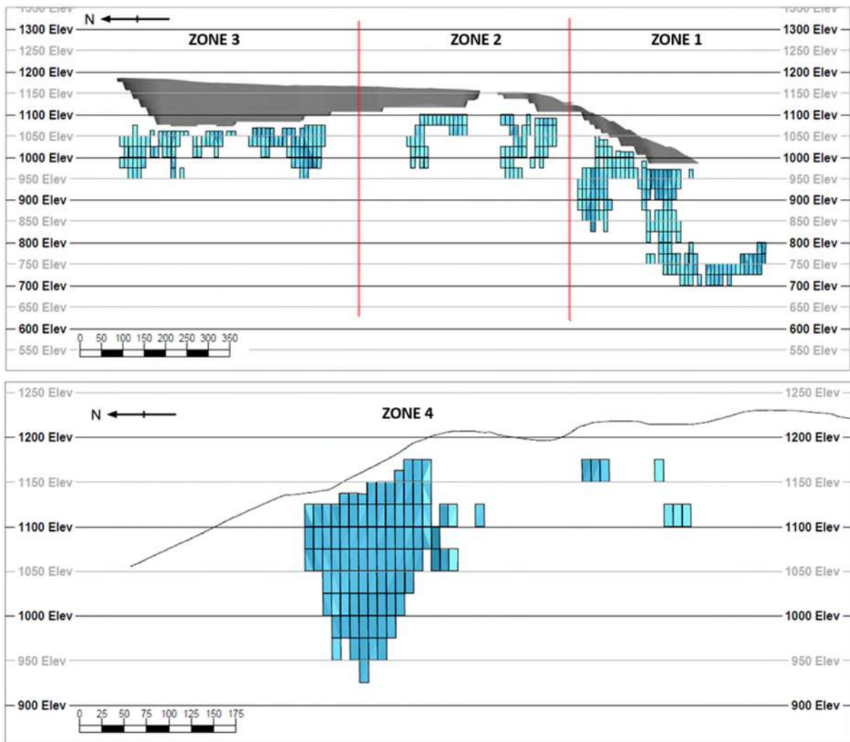
Figure 16.18: Vertikalny Stopes
